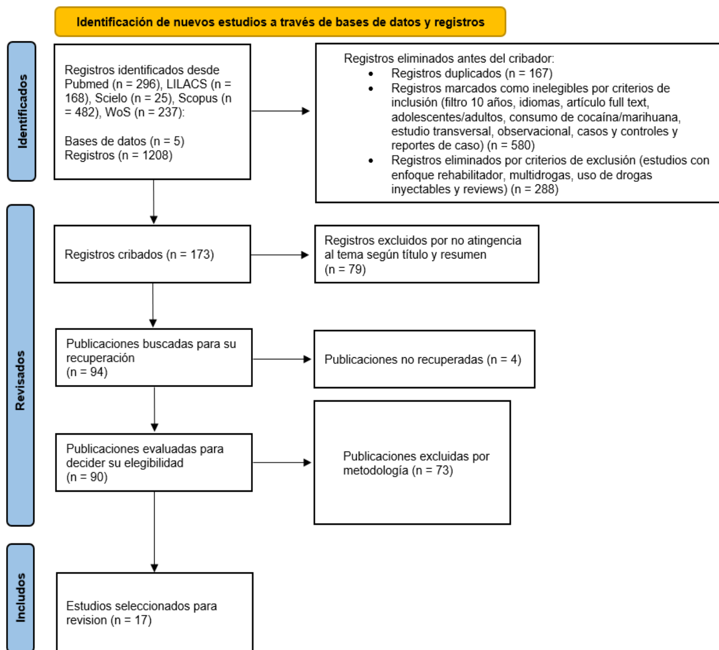
FIGURA 1 Diagrama de flujo PRISMA 2020
